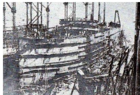
(FIG-4) “来福丸”急速建造 (起工後 11 日目)
